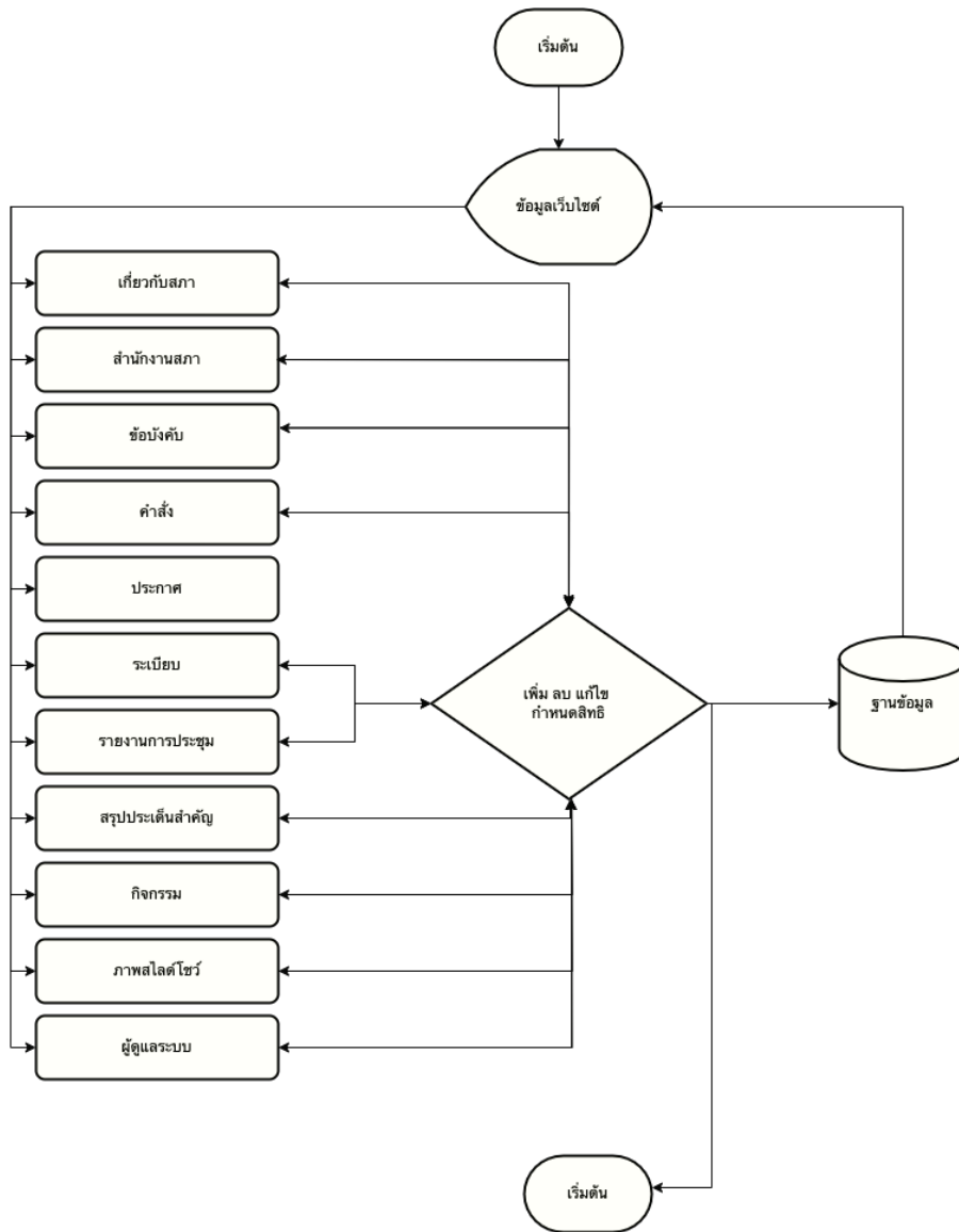
รูป Flow Chart การทำงานของระบบในส่วนของผู้ดูแลระบบ
