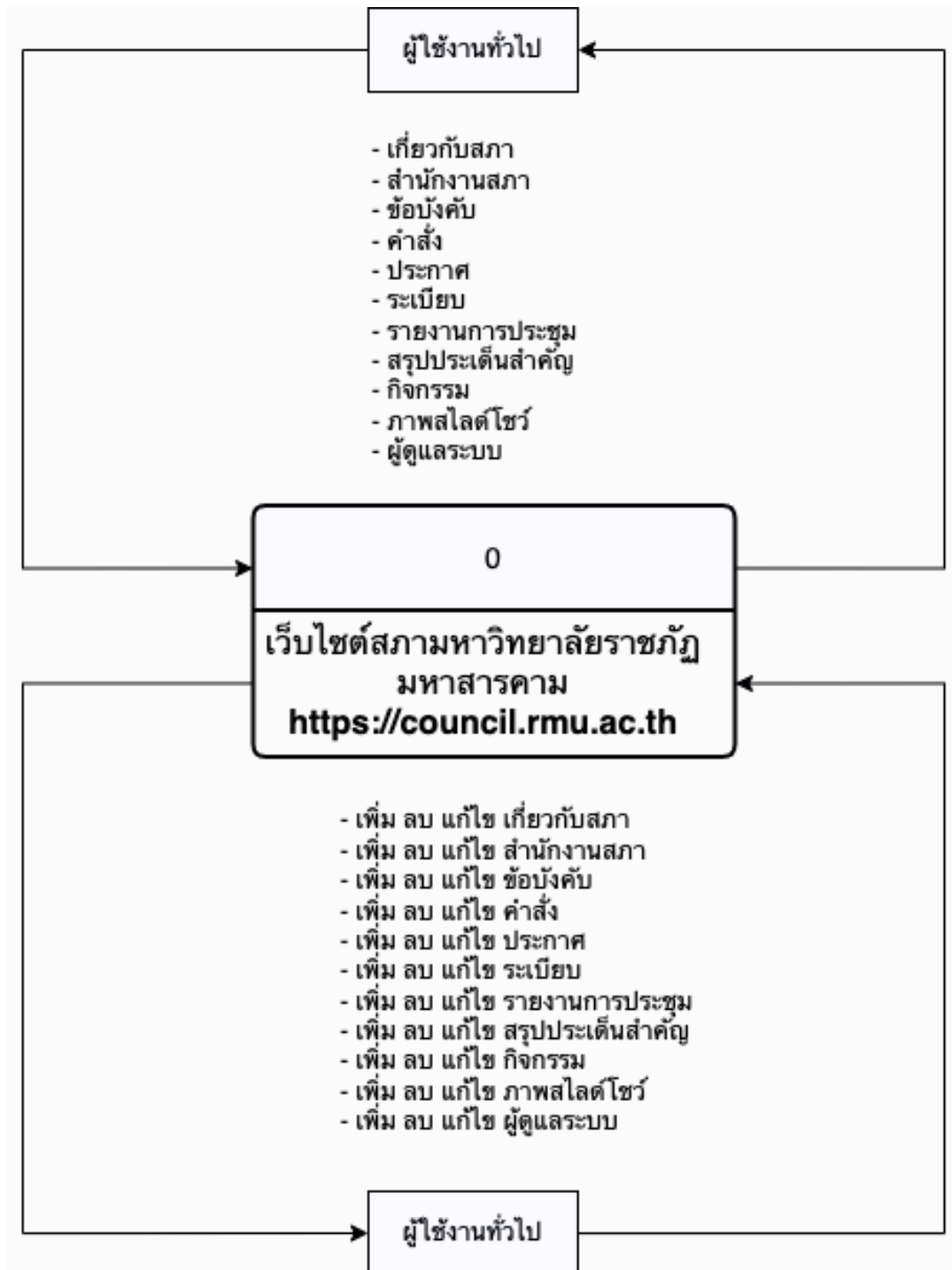
รูป Context Diagram เว็บไซต์สภามหาวิทยาลัยราชภัฏมหาสารคาม
